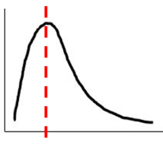
Assimetria positiva Mediana < Média
