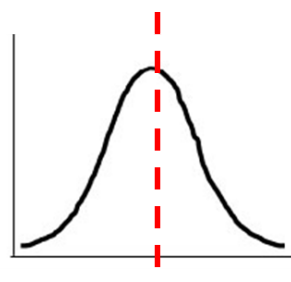
Distribuição normal Mediana ≈ Média
